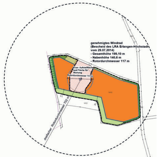
Abb. Bebauungsplan
